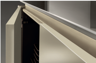
GOLA IN ALLUMINIO LACCATO LUCIDO O OPACO NEI COLORI LACCATI GLOSSY OR MATT LACQUERED ALUMINIUM RECESSED GRIP PROFILE IN THE LACQUERED COLOURS. GORGE EN ALUMINIUM LAQUÉ BRILLANT OU MAT DANS LES COLORIS LAQUÉ. GRIFFRILLE AUS IN LACKFARBEN MATT ODER HOCHGLANZ LACKIERTEM ALUMINIUM. GOLA EN ALUMINIO LACADO BRILLO O MATE EN LOS COLORES LACADOS. ПАЗ ИЗ АЛЮМИНИЯ С ЛАКИРОВАННОЙ ГЛЯНЦЕВОЙ ИЛИ МАТОВОЙ ОТДЕЛКОЙ В ЦВЕТАХ ЛАКИРОВАННЫХ ОТДЕЛОК. 采用烤漆颜色的亮光或哑光喷漆铝把手槽
